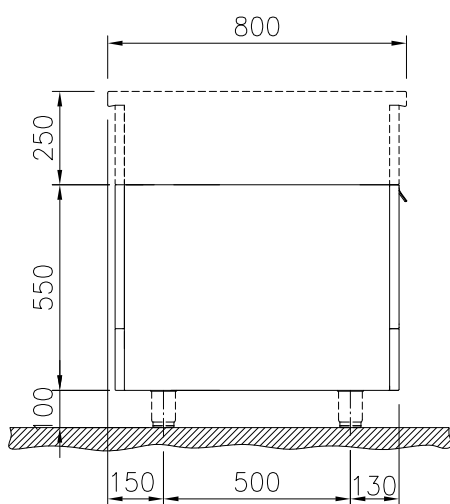
Boven aanzicht
